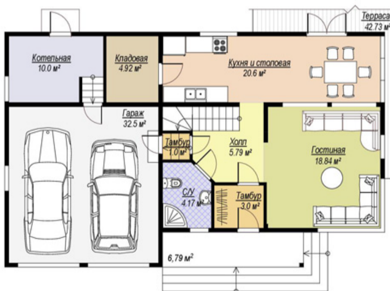
ПЛАН 1 ЭТАЖА
