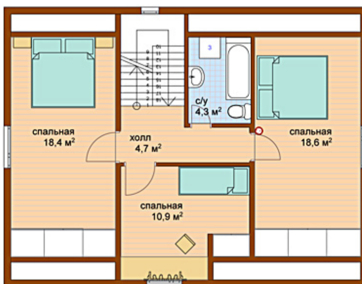
ПЛАН 2 ЭТАЖА
